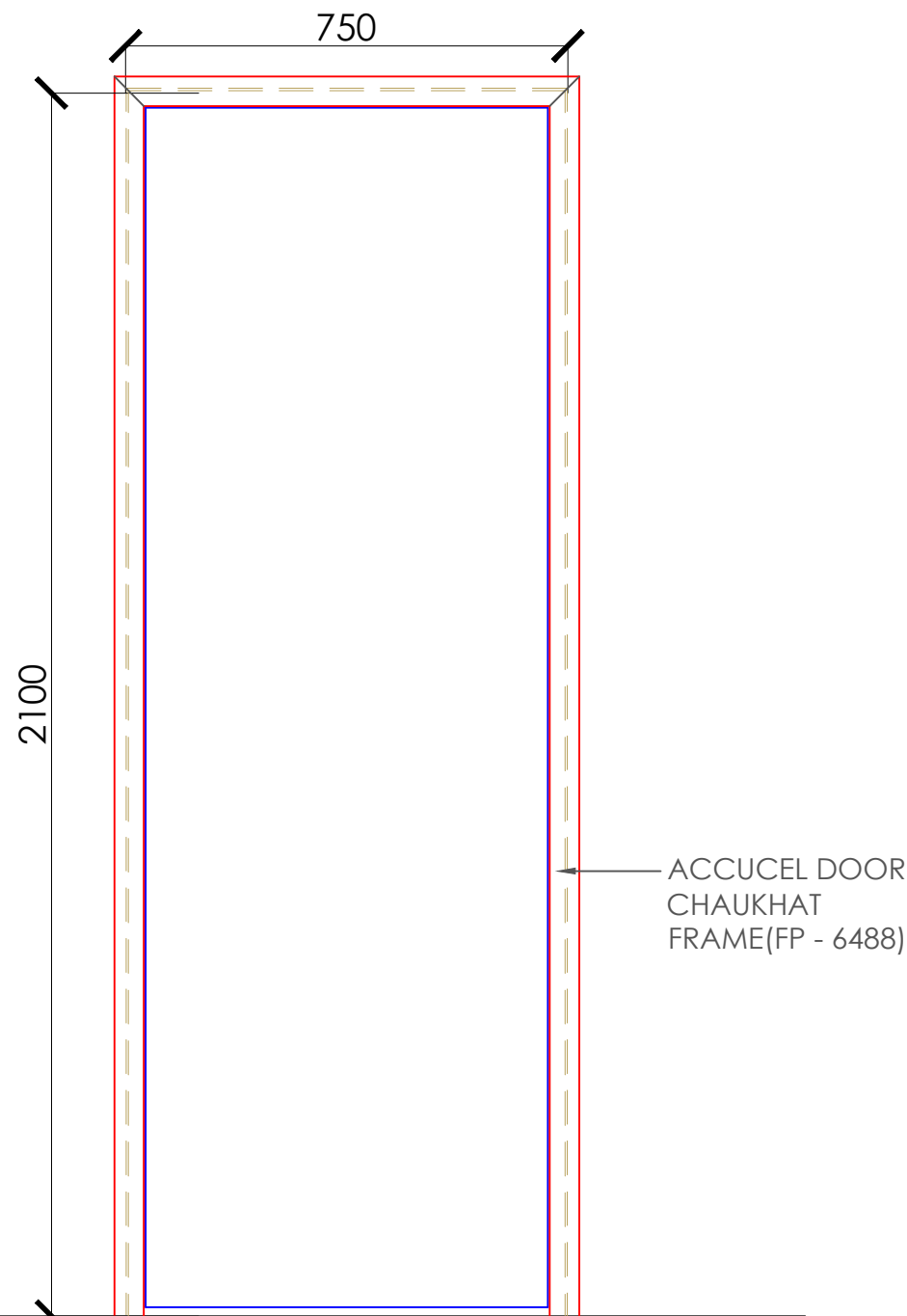
FRAME ELEVATION
